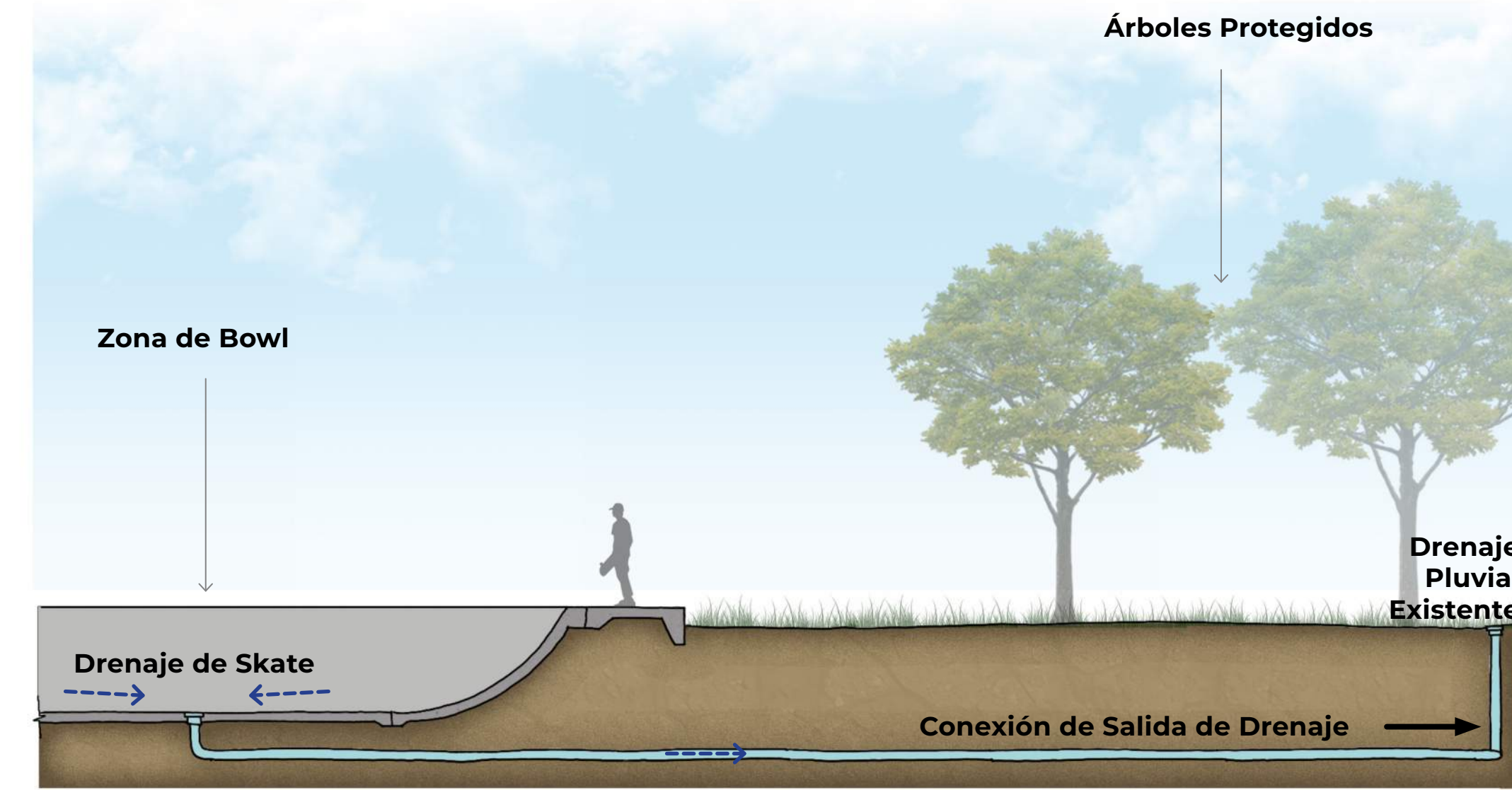
CONCEPTO DE LÍNEA DE DRENAJE 1
