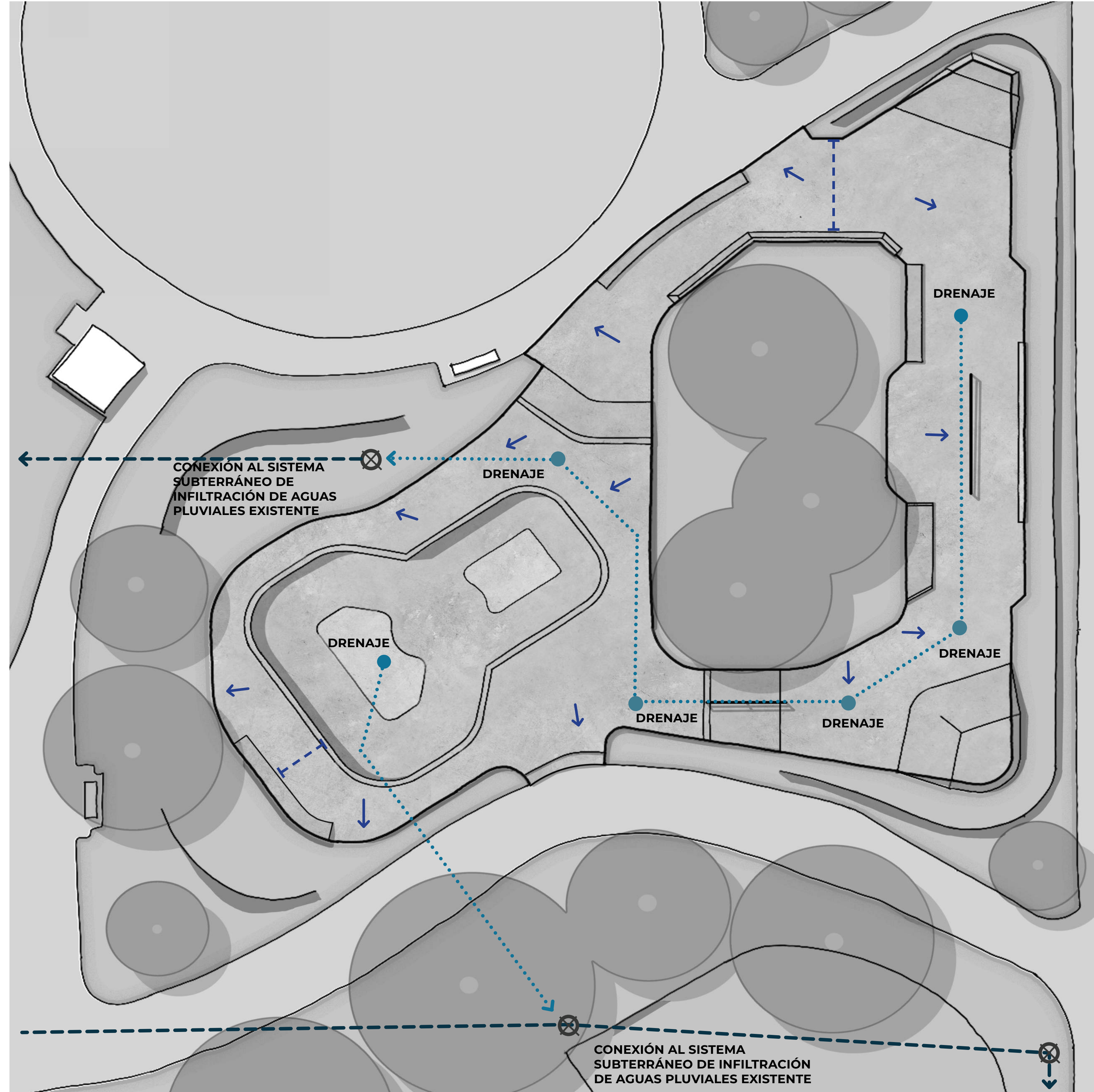
CONCEPTO DE LÍNEA DE DRENAJE 1
