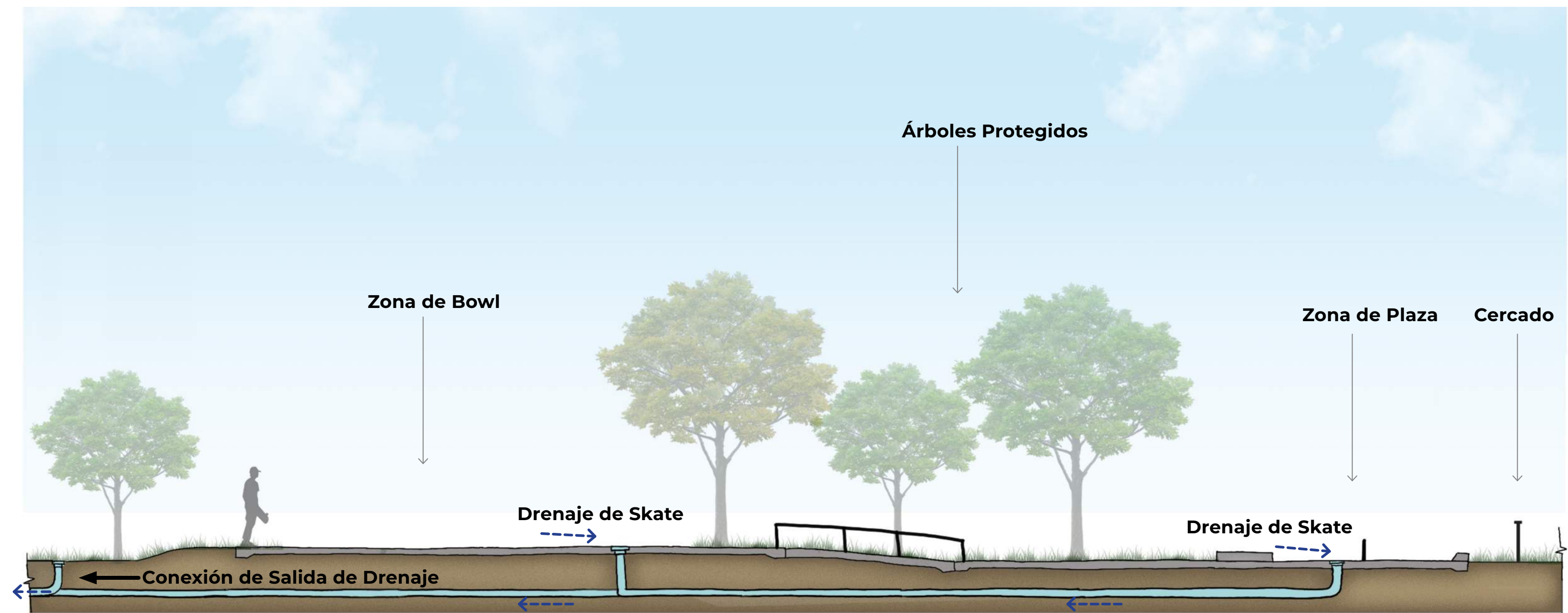
CONCEPTO DE LÍNEA DE DRENAJE 2
